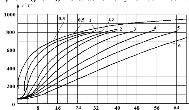
Рисунок 2 – Залежність температури сталі від приведеної товщини перерізу (см) та часу нагрівання за стандартним температурним режимом
