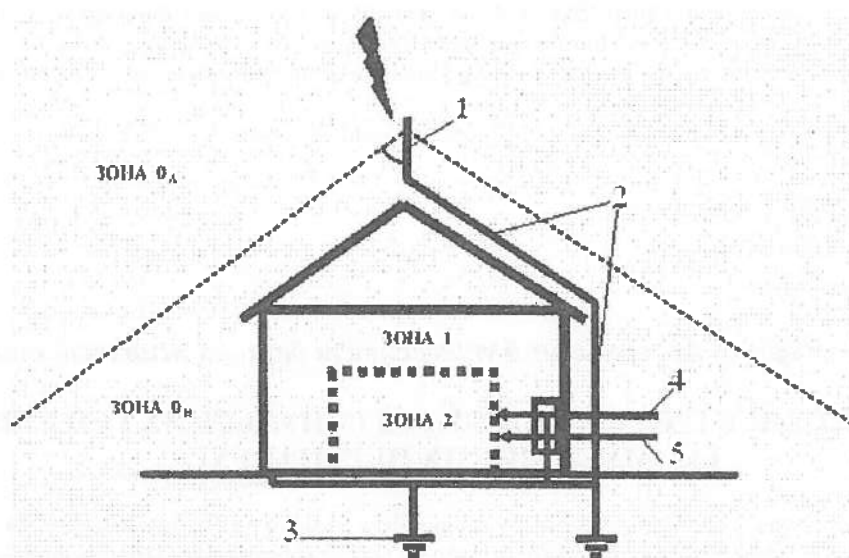
Рис. 1. Схема зон блискавкозахисту з погляду прямої і непрямой дії блискавки 1 – блискавкоприймач, 2 – струмовідвід, 3 – заземлювач, 4 – електричні і 5 – неелектричні комунікації
