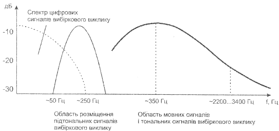
Рис. 1. Границі розміщення сигналів вибіркового виклику
