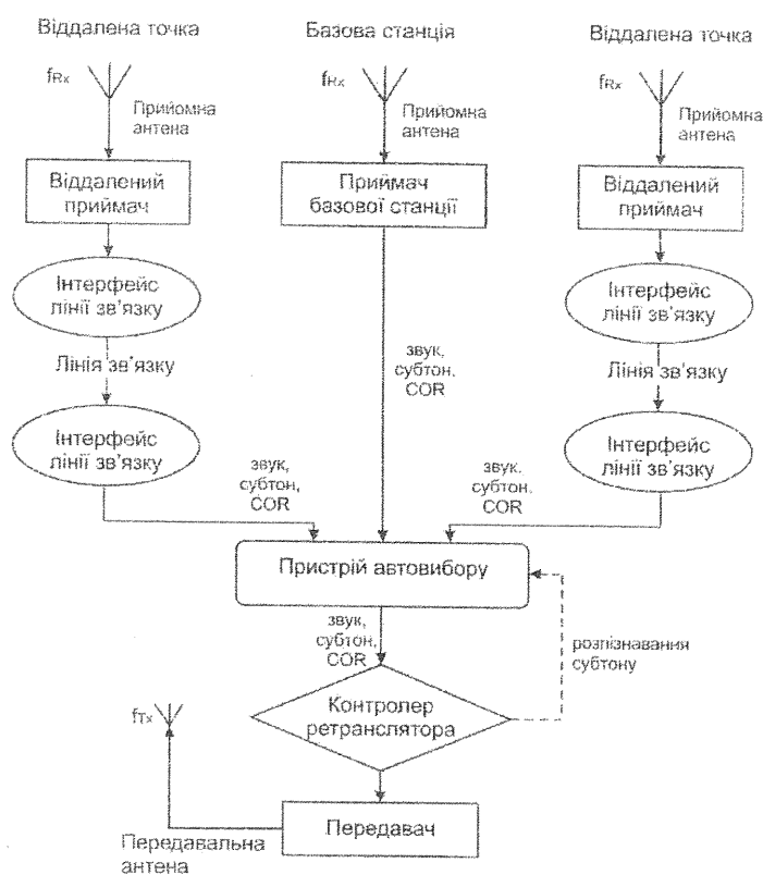
Рис. 3. Принцип організації системи віддаленого прийому
