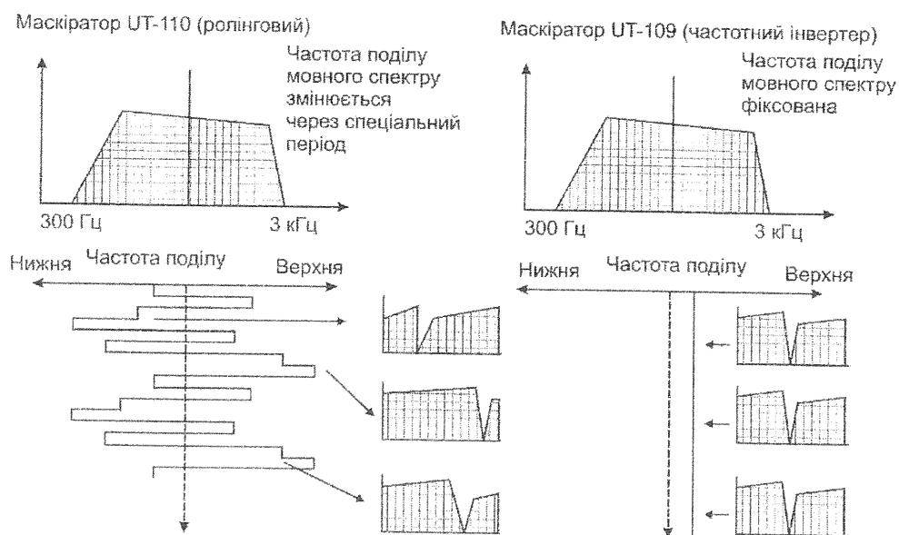
Рис. 2. Схема перетворень мовного сигналу в часі в маскіраторах на прикладі скремблерів Icom UT-109 та UT-110
