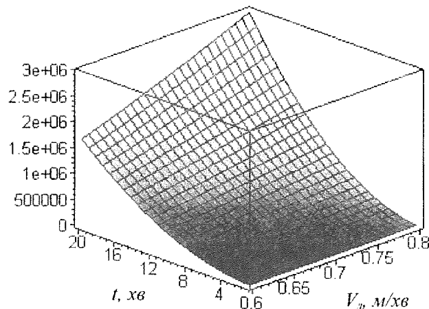
Рис. 1. Кількість енергії, яка виділяється під час горіння горючого навантаження квартири за хвилину Q_{вид} , протягом часу розвитку пожежі t при заданій лінійній швидкості поширення полум'я V_p
