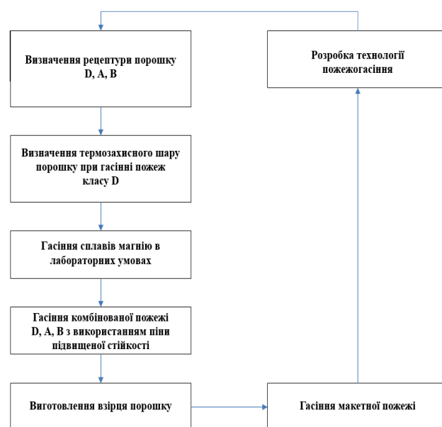
Рисунок 1 – Алгоритм дослідження
