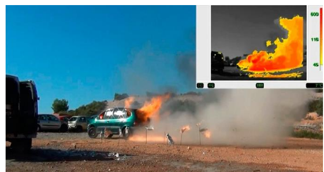
Рисунок 3 – Приклад горіння водню в АВП та його зображення на моніторі пожежного тепловізора
