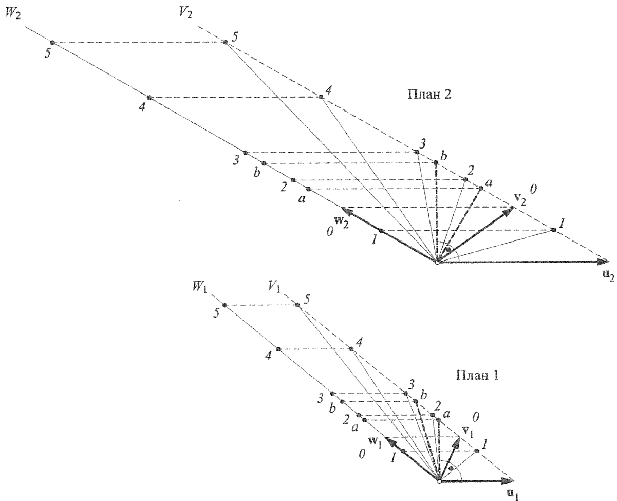
Рисунок 4 — Плани швидкостей руху плинної речовини на різних режимах роботи ідеальної помпи
