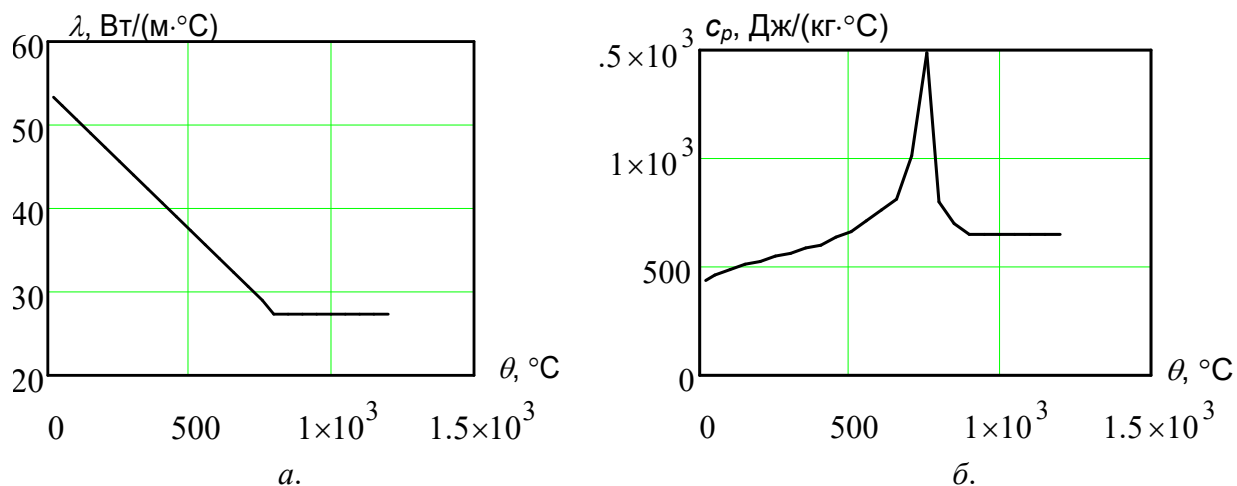
Рисунок 7 – Теплофізичні характеристики сталеві обійми тубобетонної колони: а – коефіцієнт теплопровідності; б – питома теплоємність
