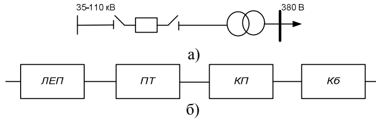
Рис. 4. Схеми електроживлення: а) принципова; б) логічна
