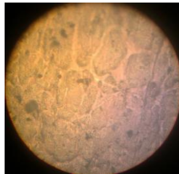
Рис.5. Мікроструктура мідного дроту після пропускання струму I = 400 А, протягом 10 с і дії відкритого полум'я t = 582 °С протягом 15 хв: а – травник №1 \times 200 ; б – травник №2 \times 500
