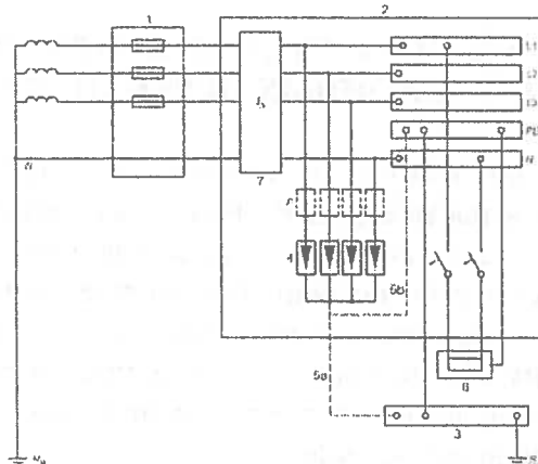
а) Установлення ПЗІП на межі зон 0_A/1 ( 0_B/1 ) в системах заземлення TN
