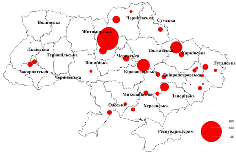
Рисунок 2 – Результати оцінювання емісій парникових газів при спалюванні природного газу для виробництва електроенергії в Україні в CO 2 -еквіваленті (2012 р., тис. т)
