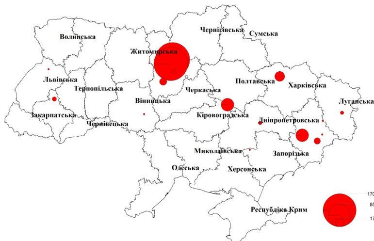
Рисунок 3 – Результати оцінювання емісій парникових газів при спалюванні мазуту для виробництва електроенергії в Україні в CO 2 -еквіваленті (2012 р., тис. т)
