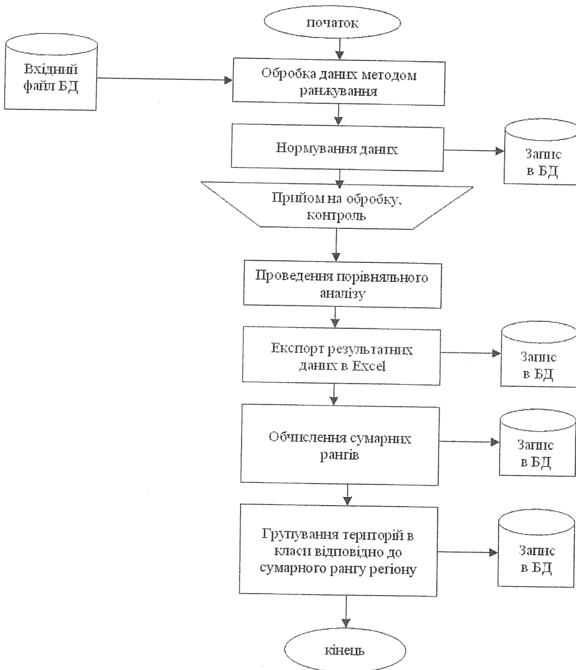
Рис. 1. Узагальнена блок-схема оцінки екологічного стану регіонів України
