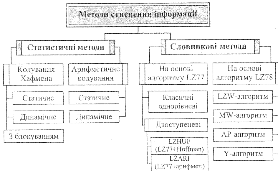
Рис. 1. Класифікація методів стиснення інформації
