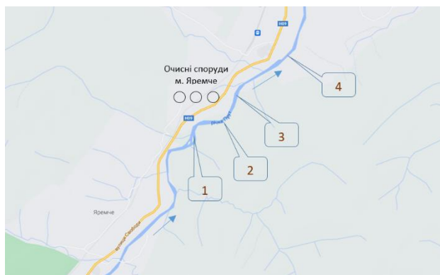
Рисунок 1 – Схема району досліджень та точок відбору проб донних відкладень
