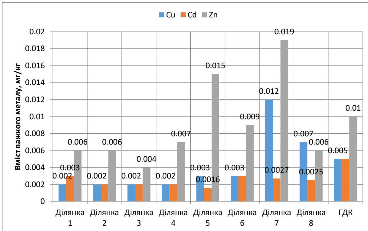
Рисунок 1 – Вміст важких металів у воді ріки Стир
