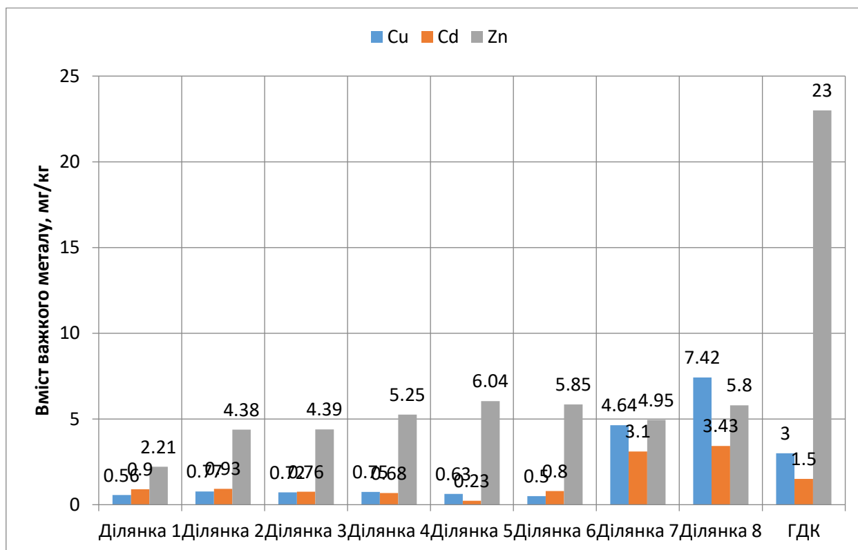
Рисунок 2 – Вміст важких металів у едафотопах прибережної зони річки Стир
