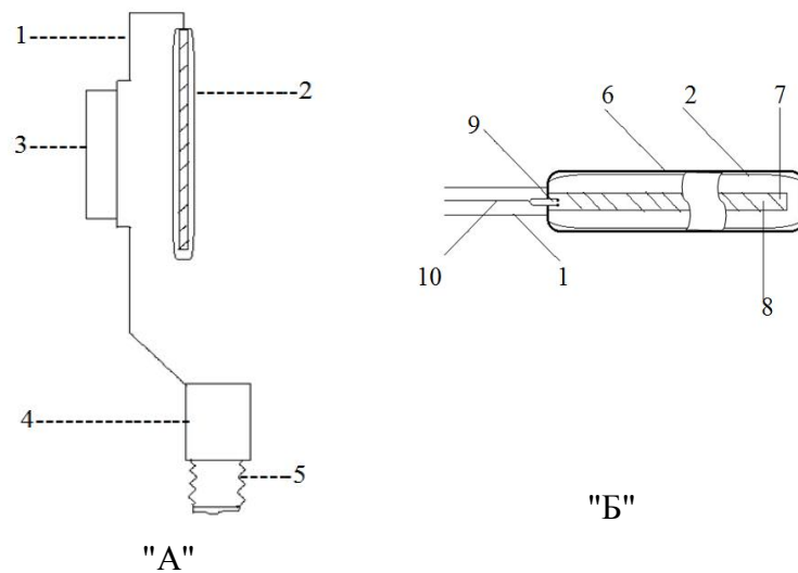
Рис. 3. Схема енергорекупераційного апарата для ламп освітлення та схема мультиферронового тепло-електрорекуператора.
