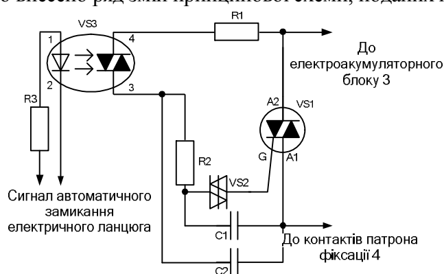
Рисунок 8 – Принципова схема електронного комутаційного пристрою автоматичного керування енергорекуперативним апаратом
