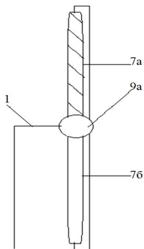
Рис. 5. Схема мультиферронового теплоелектрорекуператора: 7а, 7б – термоелектроди; 9а – електродна точка
