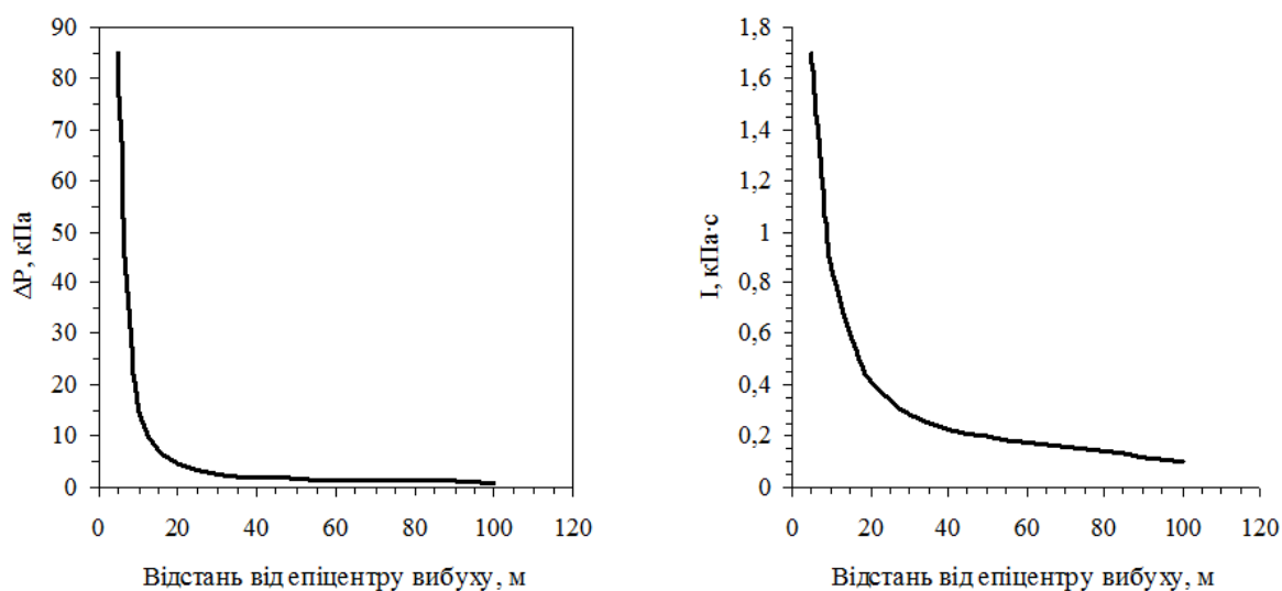
Рис. 2. Зміна уражаючих чинників вибуху кисневого балона залежно від відстані до епіцентру вибуху
