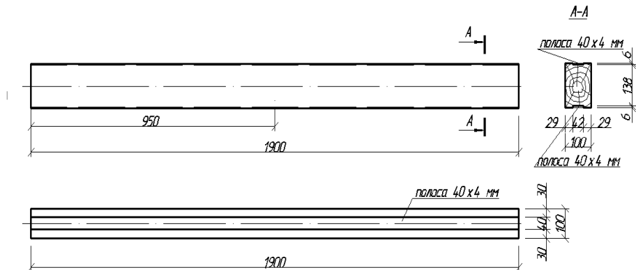
Рис. 2. Схема армування дослідних зразків серії II та IV
