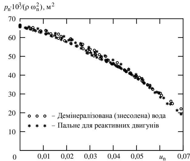
Рис. 8. Ідентифікація автотомельності режимів роботи відцентрової помпи (Hale Products Inc., США)
